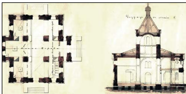
Проект церкви, предполагаемой постройкой в с. Обдорском. Российский государственный исторический архив
